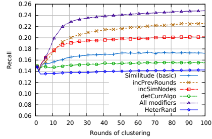
Fig. 16. Recall (MovieLens)
